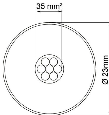
Leitungsquerschnitt
