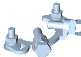
Mastsicherung
