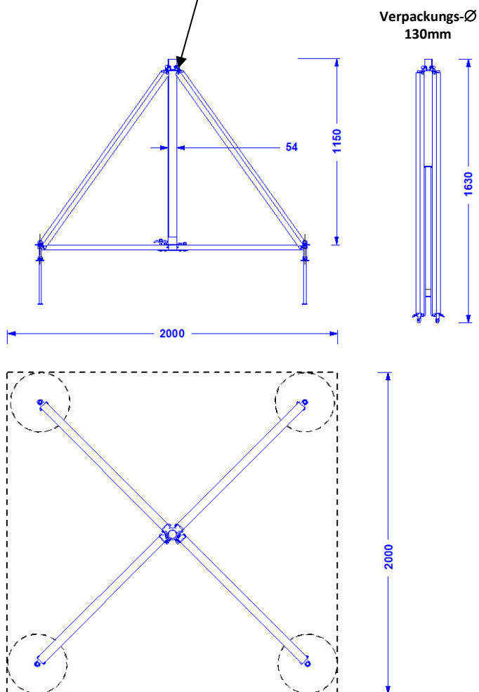
Mastsicherung
