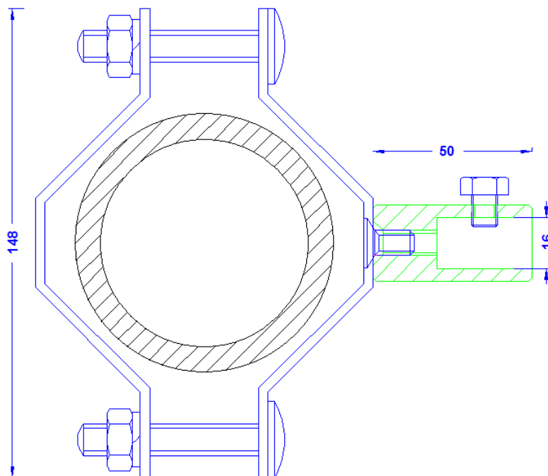
Front - Schnitt
