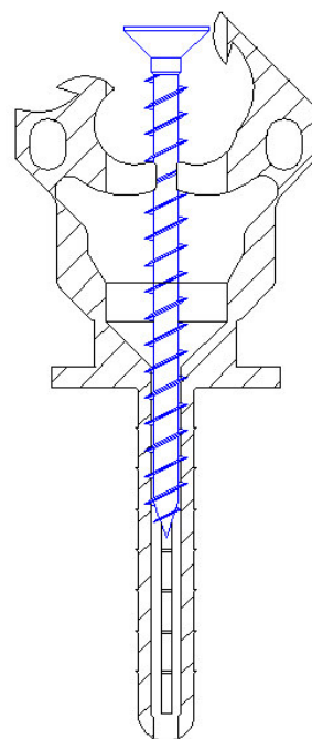
Schnitt
