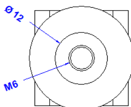
Unten
