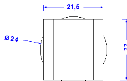
Oben
