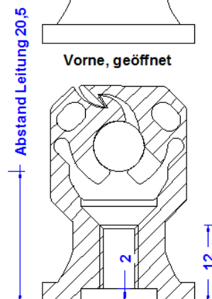
Schnitt
