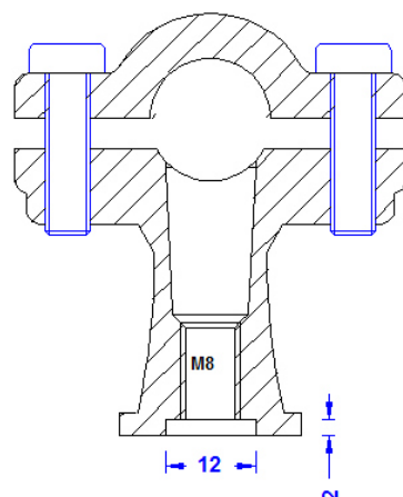
Schnitt
