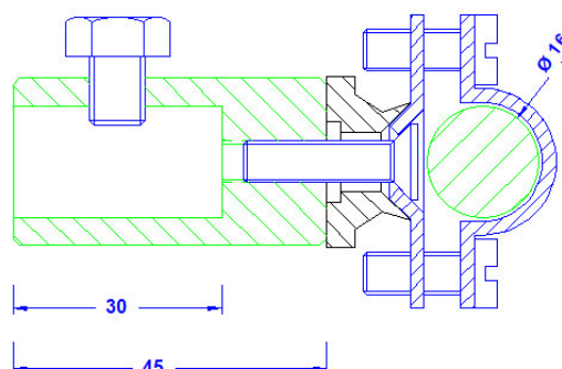
Front - Schnitt
