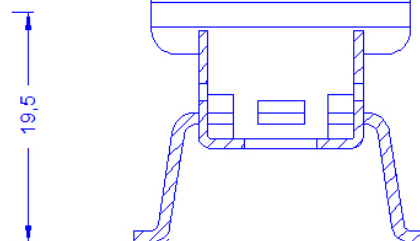
Schnitt
