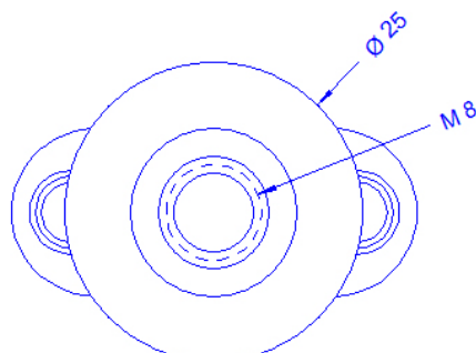
Unten
