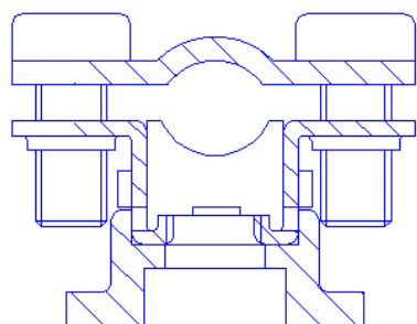
Schnitt
