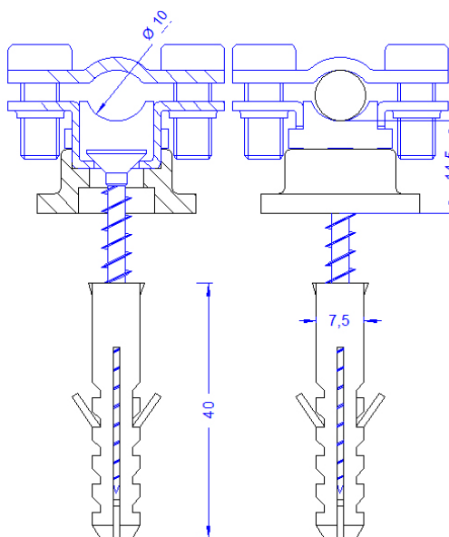
Schnitt
