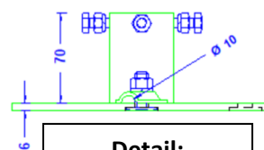
Detail: Grundplatte
